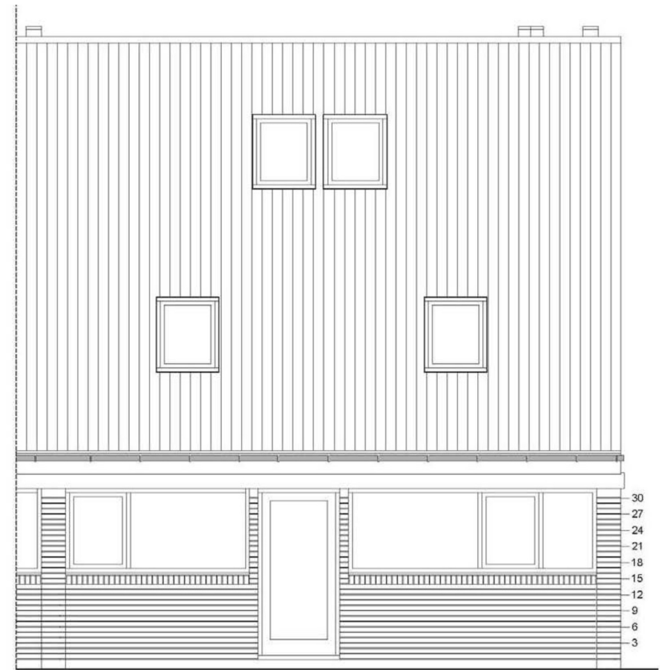
Facade Øst
